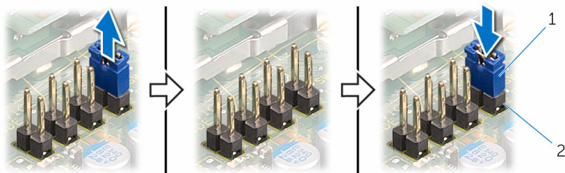
1 跳线塞
